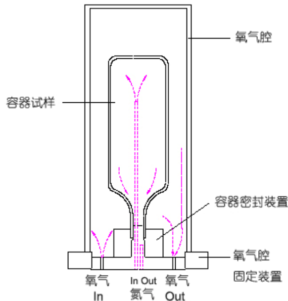
图 2. TOY-C1 包装容器固定方式示意图
